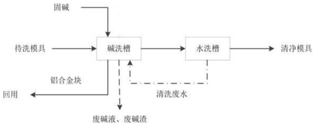
3.4-7 碱洗间工艺流程及产物节点图
