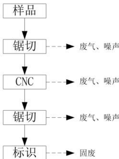
3.4-2 型材拉伸样工艺流程及产物节点图
