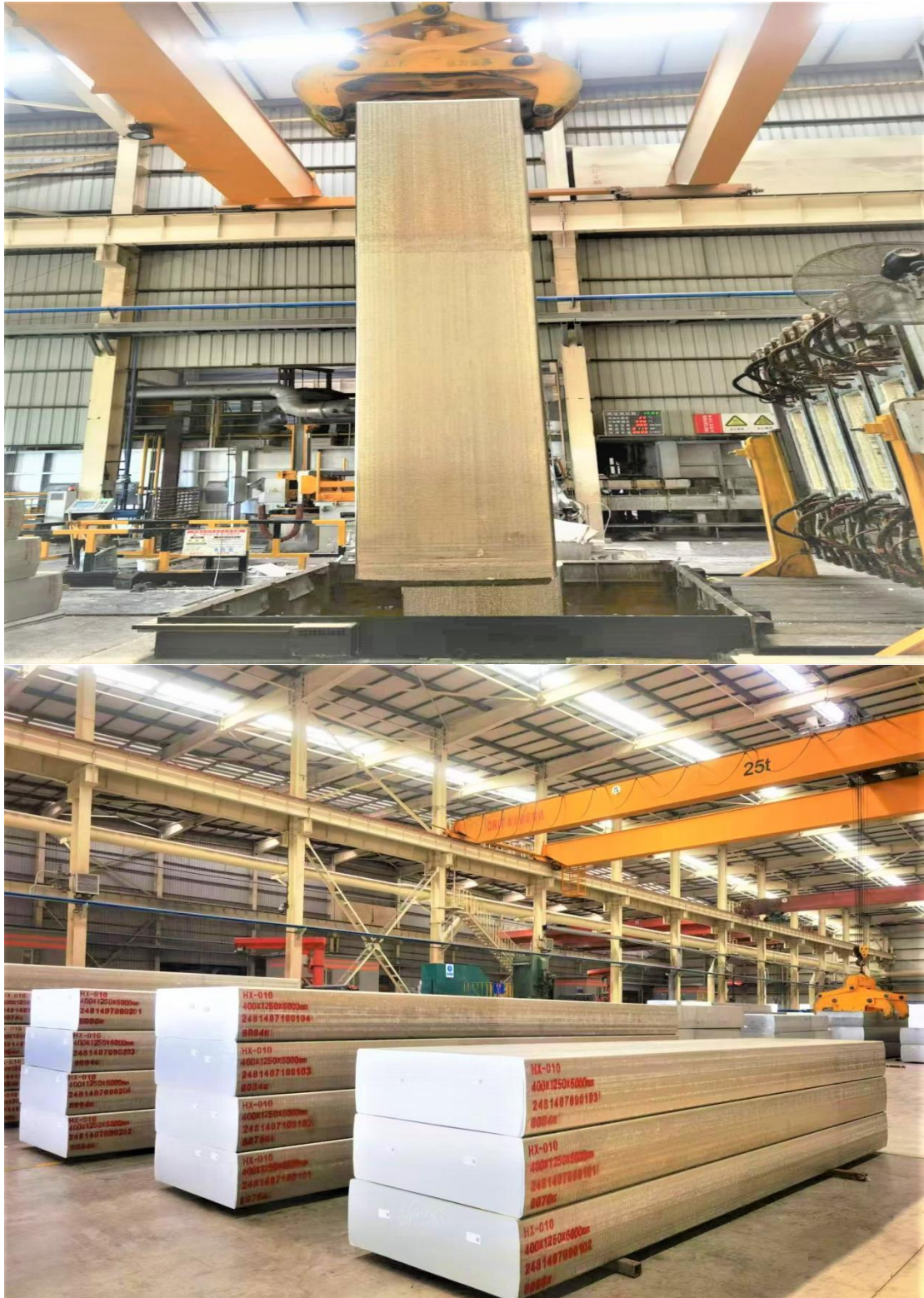
图 1-5 铝扁锭图
